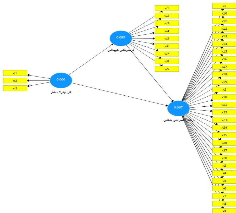
شکل ۳: نمودار بررسی اعتبار حشو یا افزونگی مدل
