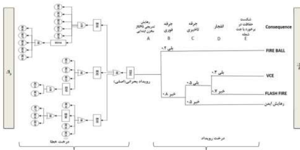
شکل ۴: دیاگرام Bowtie مربوط بہ رہایش تدریجی گاز LPG
